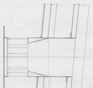
DETALLE SECCION 5-5 - ESCALA NATURAL
