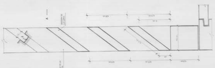
DETALLE SECCION DE PARTES DE LA GARITA 1-1 - ESCALA NATURAL
